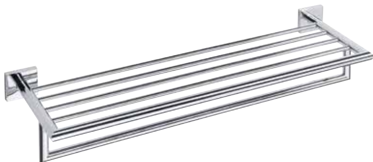
■ Držák ručníků Towel holder | Handtuchhalter Полотенцедержатель 132204012 355 x 55 x 65 mm 132204022 505 x 55 x 65 mm 132204042 655 x 55 x 65 mm
