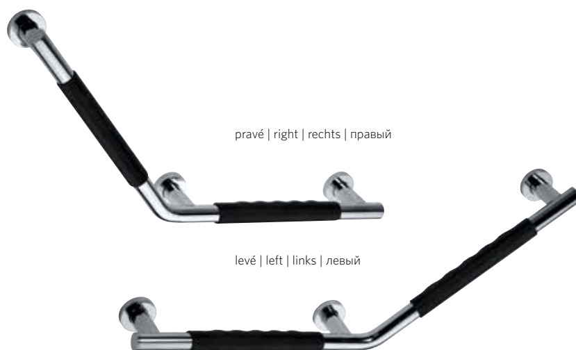
Madlo 135°, guma 135° grab bar, black rubber Wannengriff abgewinkelt 135°, schwarze Gummi Поручень изогнутый 135°, черная резина 715 x 325 x 80 mm 104507711 pravé | right | rechts | правый 104507701 levé | left | links | левый
