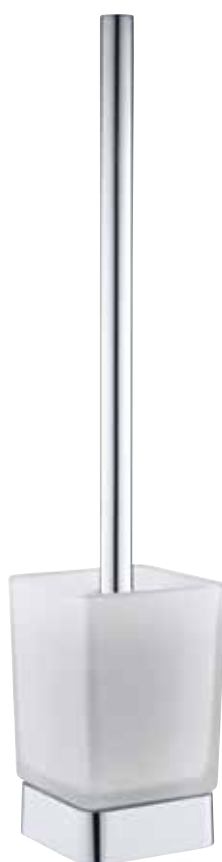
■ WC štětka, miska sklo Wall mounted toilet brush with glass WC-Bürstengarnitur mit Glasbehälter Ёршик подвесной (стекло) 75 x 344 x 87 mm 139113142
